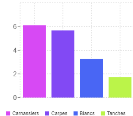
Coefficient d'accroissement/espèce
